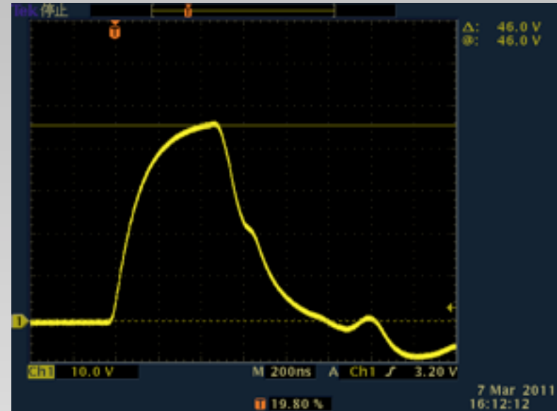
20Ω 2-turn(2.4uH)
